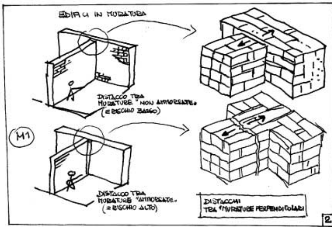
Figura 2 - Distacchi tra "murature perpendicolari"
